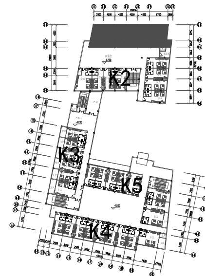
平面索引图
