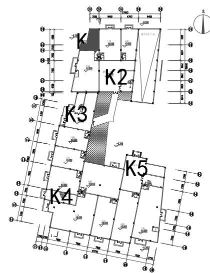
平面索引图
